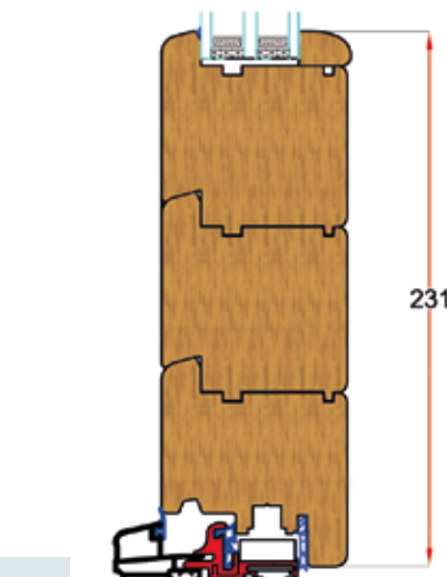
SEZIONE VERTICALE PORTAFINESTRA
