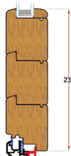
SEZIONE VERTICALE PORTAFINESTRA
