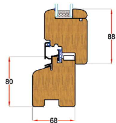
SEZIONE VERTICALE FINESTRA
